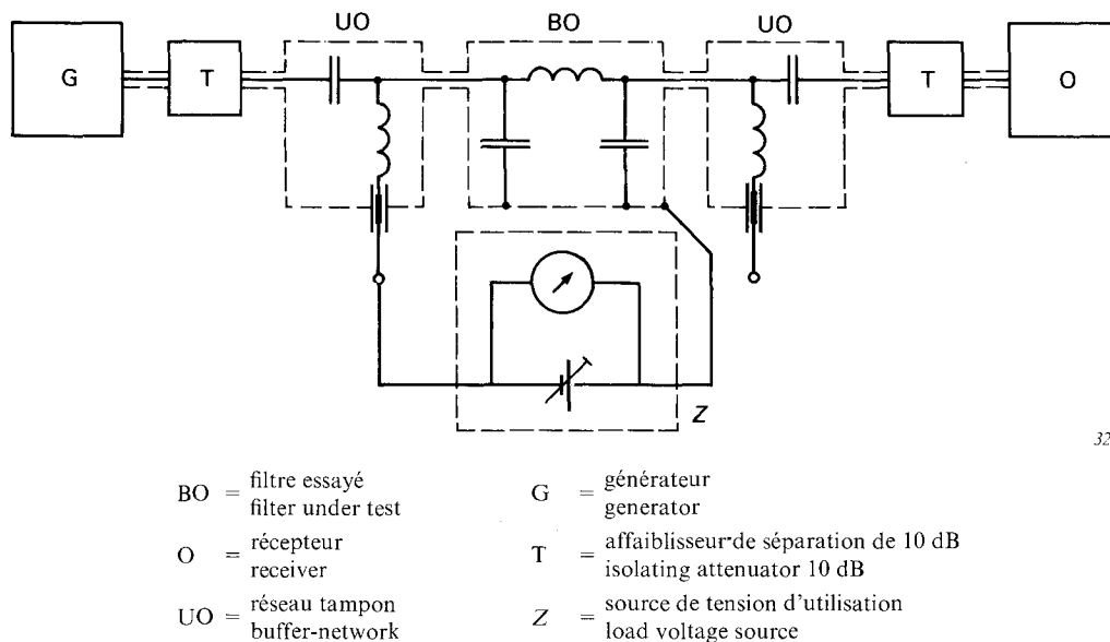
FIG. B4. — Exemple de branchement de réseaux tampons pour une source de tension d'utilisation dans un circuit de contrôle asymétrique.
