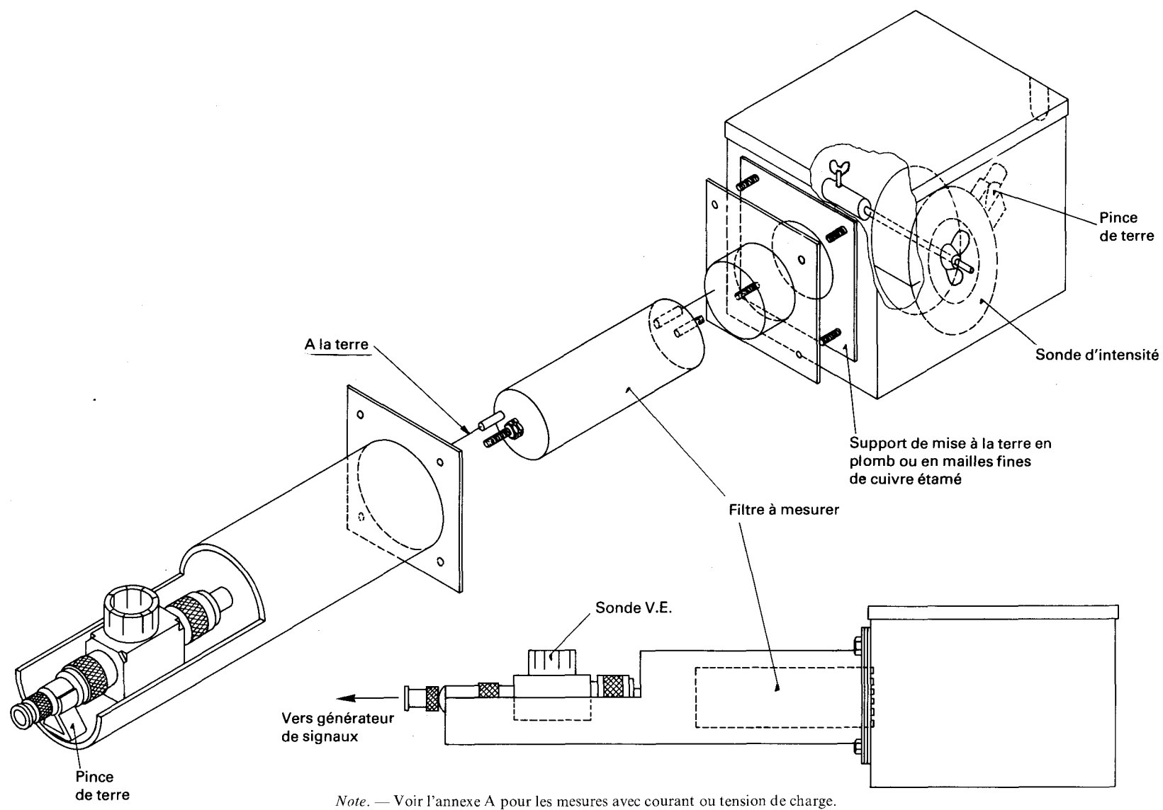
FIG. 3. — Exemple de méthode de blindage pour la mesure de l'impédance de transfert.
