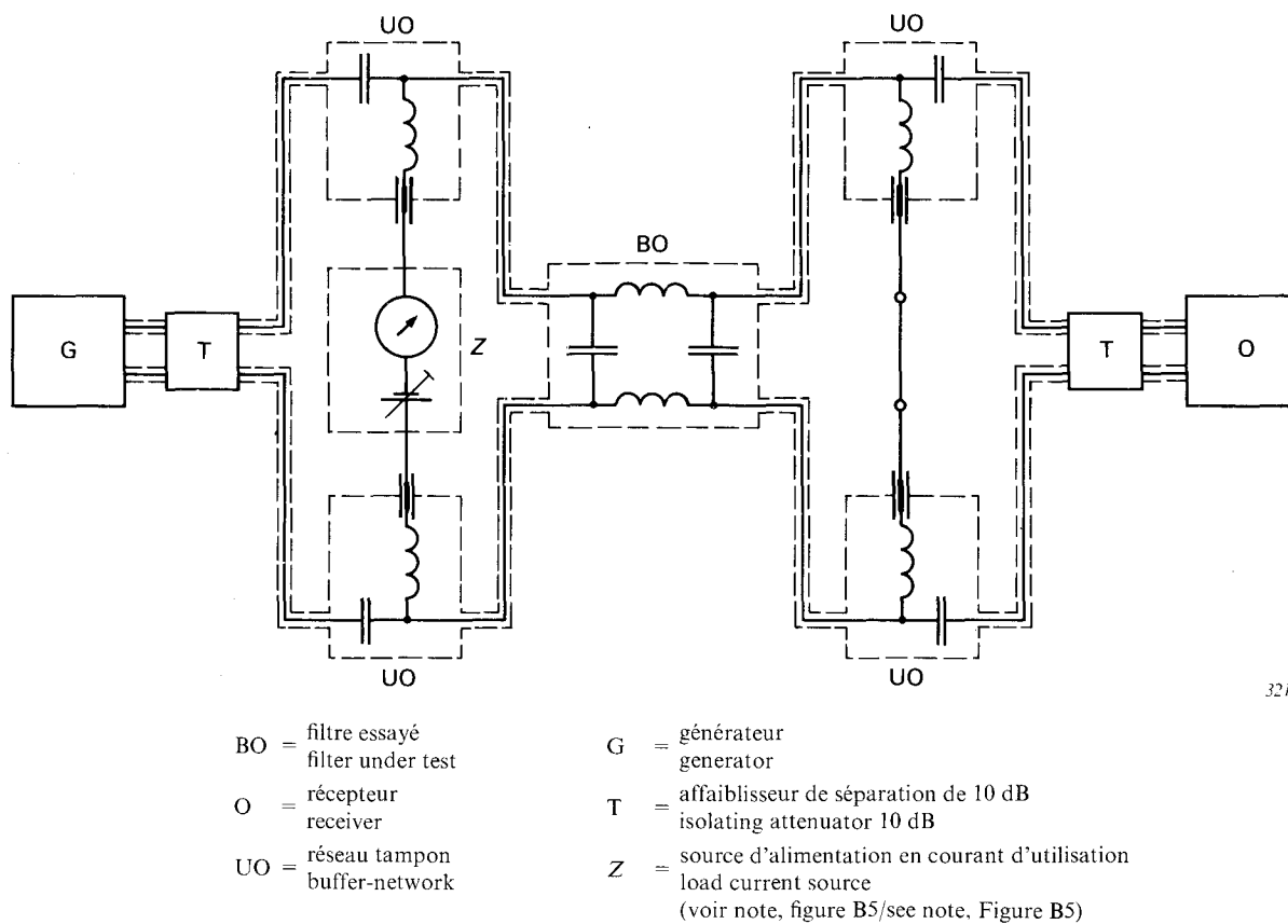
FIG. B3. — Exemple de branchement de réseaux tampons pour une source d'alimentation en courant d'utilisation, dans un circuit de contrôle symétrique.
