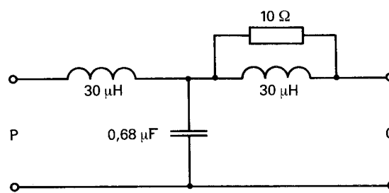
FIG. 2. — Circuit d'un filtre comprenant un amortissement résistif.
