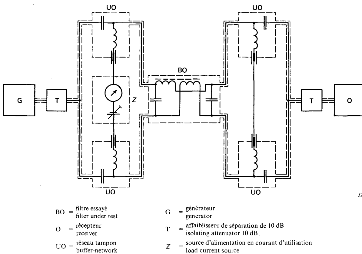
FIG. B6. — Exemple de branchement de filtre symétrique pour la mesure asymétrique de l'affaiblissement d'insertion.
