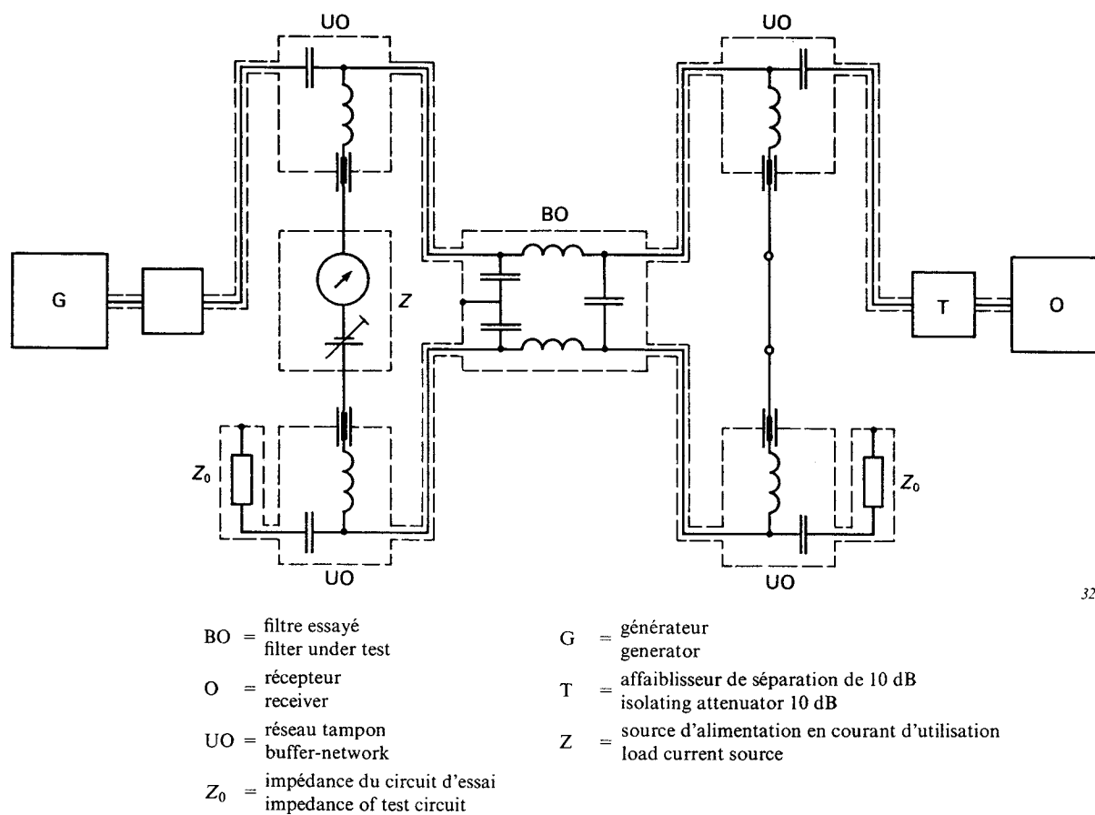
FIG. B7. — Exemple de branchement de réseaux tampons pour une source d'alimentation en courant d'utilisation dans un circuit de contrôle «V» pour filtres à deux voies. Example of connecting buffer-networks for load current source in "V" test circuit for two-line filters.
