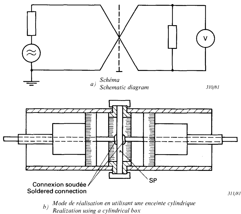
FIG. A3. — Exemple de court-circuiteur dans le circuit de contrôle. Example of short circuit in test circuit.
